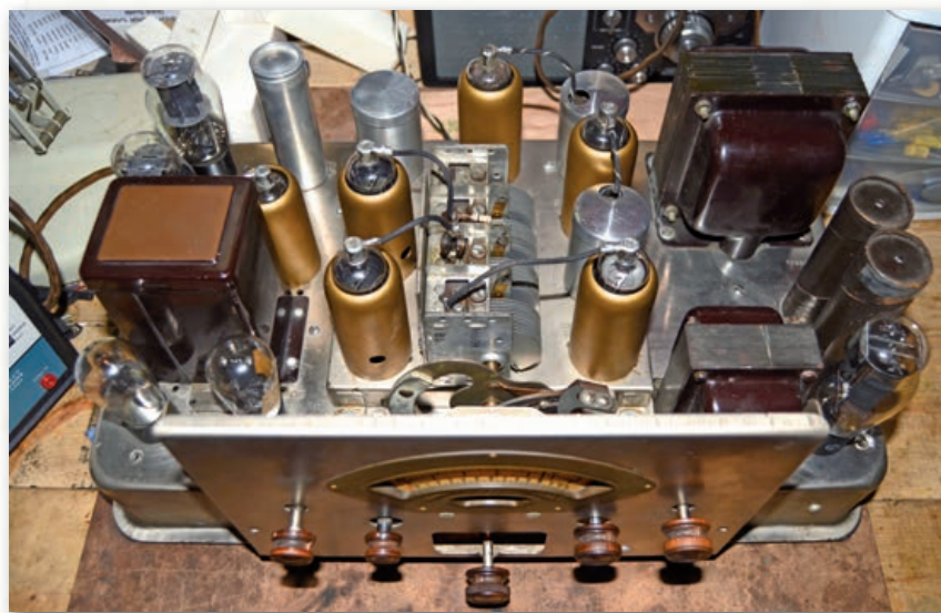
Interior de un Atwater Kent 711 restaurado
